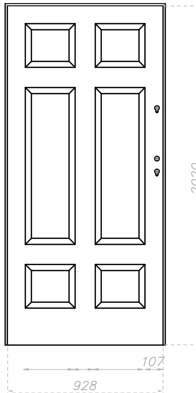
Strona przeciwna do zawiasowej
