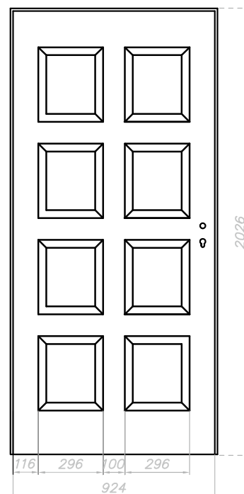
Strona przeciwna do zawiasowej
