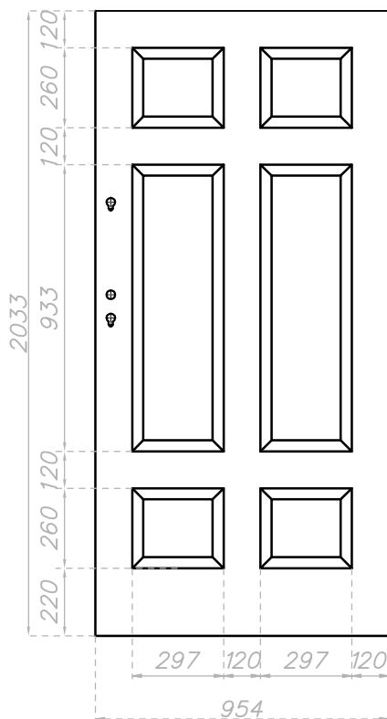
Strona zawiasowa
