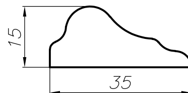
Profil listwy wystrojowej G
