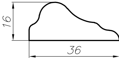
Profil listwy wystrojowej H
